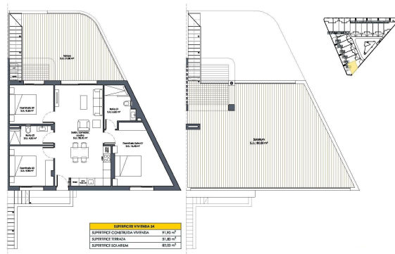
VIVIENDA 34 - PLANTA PRIMERA Y SOLARIUM
