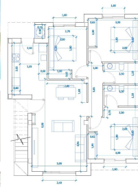
PLANTA MODELO A
